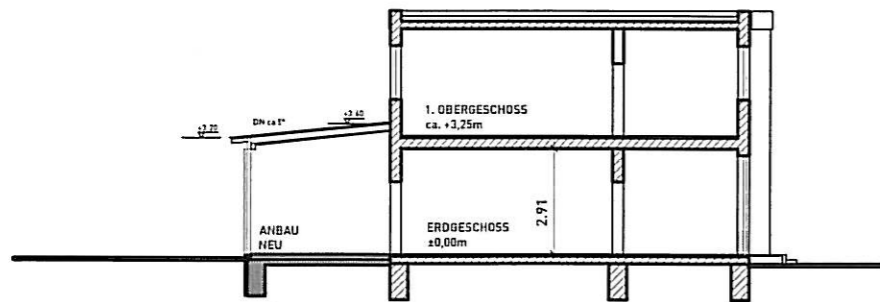
SCHNITT I-I
