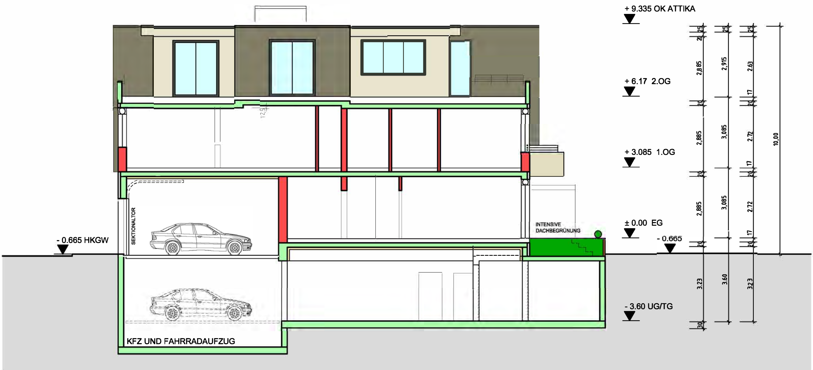
SCHNITT B-B / ANSICHT NORD-WEST
