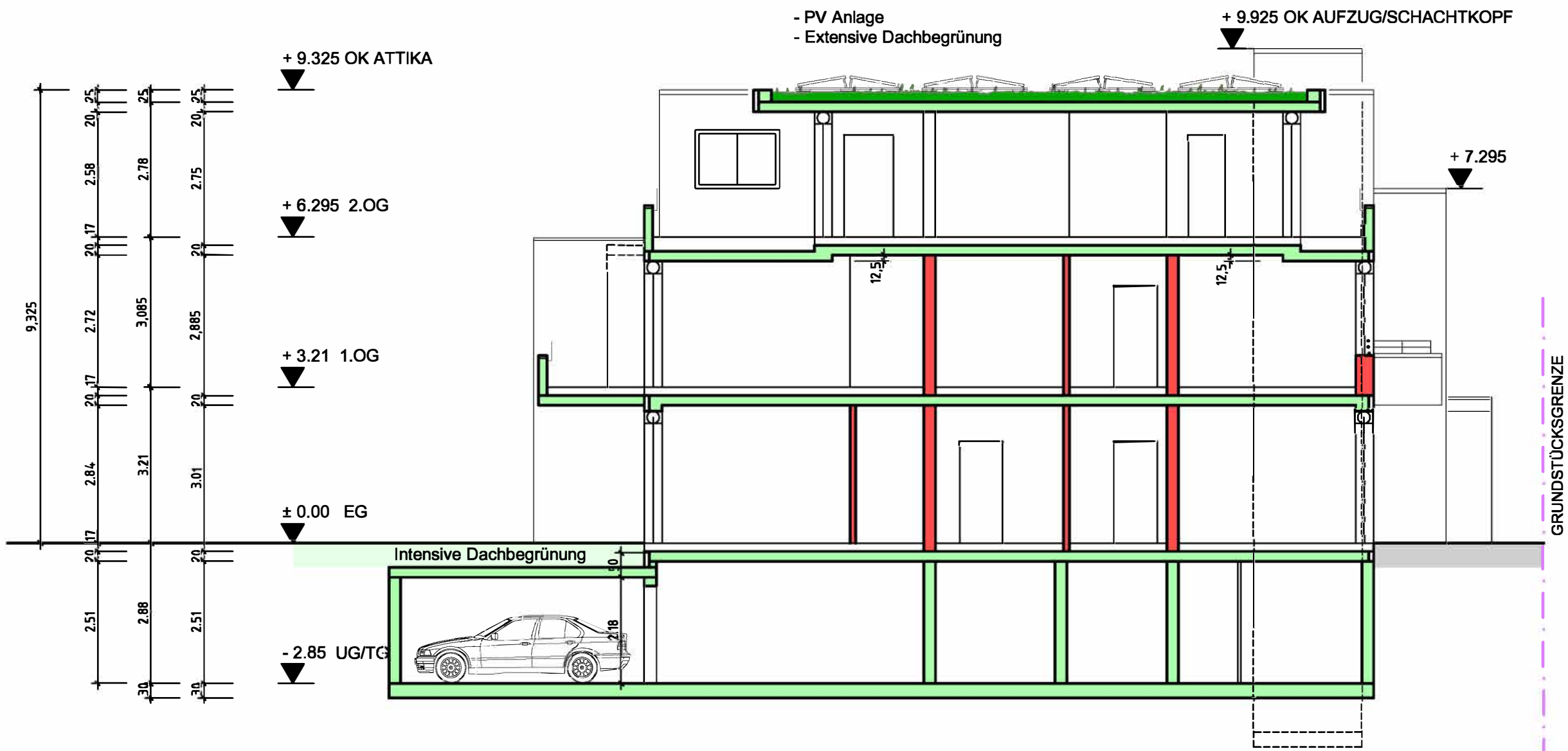
SCHNITT A-A
