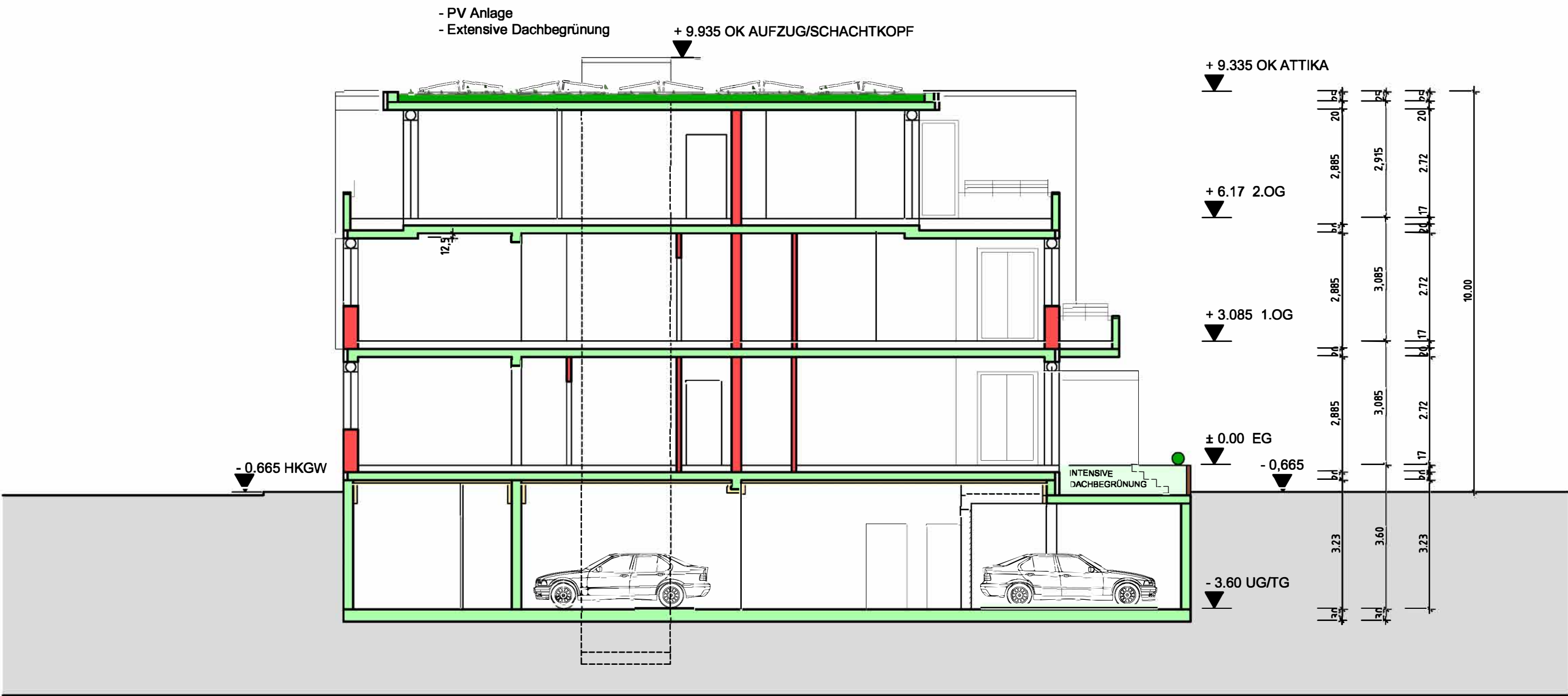
SCHNITT A-A
