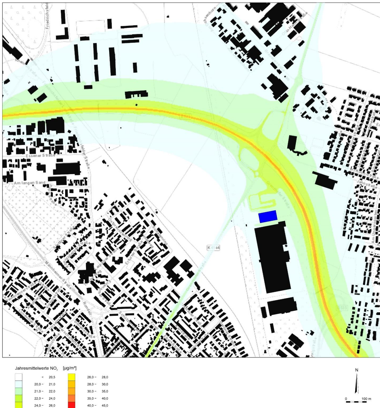
Abbildung A- 2: Jahresmittelwerte \text{NO}_2 , Planfall 2022.
