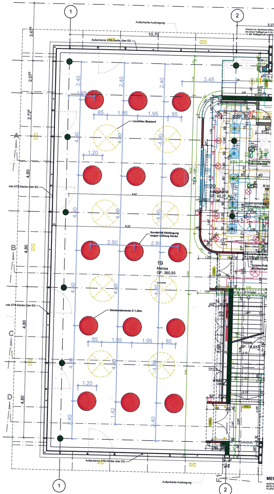
GRUNDRISS 1.OG
